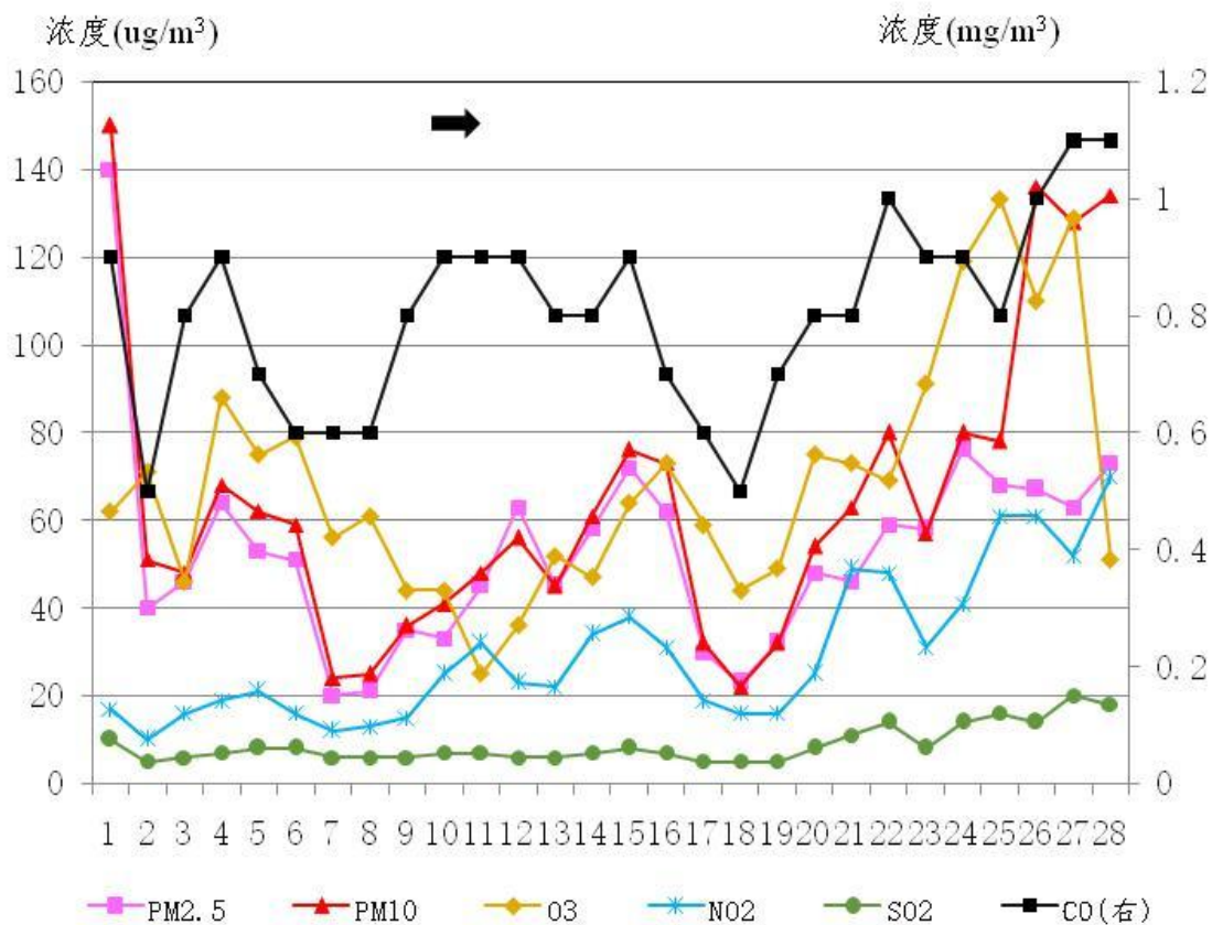
图1 2月份鄂州市城区六项污染物日浓度变化趋势
