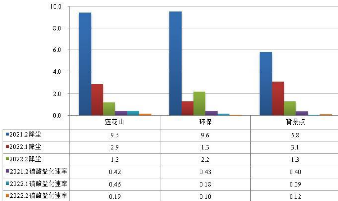
图5 城区2月降尘及硫酸盐化速率
