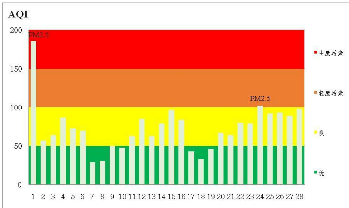
图2 2022年2月鄂州市区空气质量指数分布图
