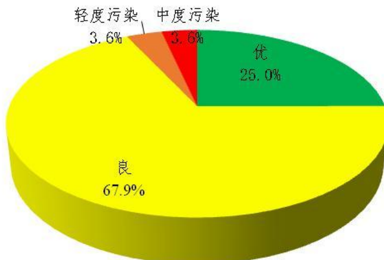
图2 2022年2月鄂州市区空气质量指数分布图
