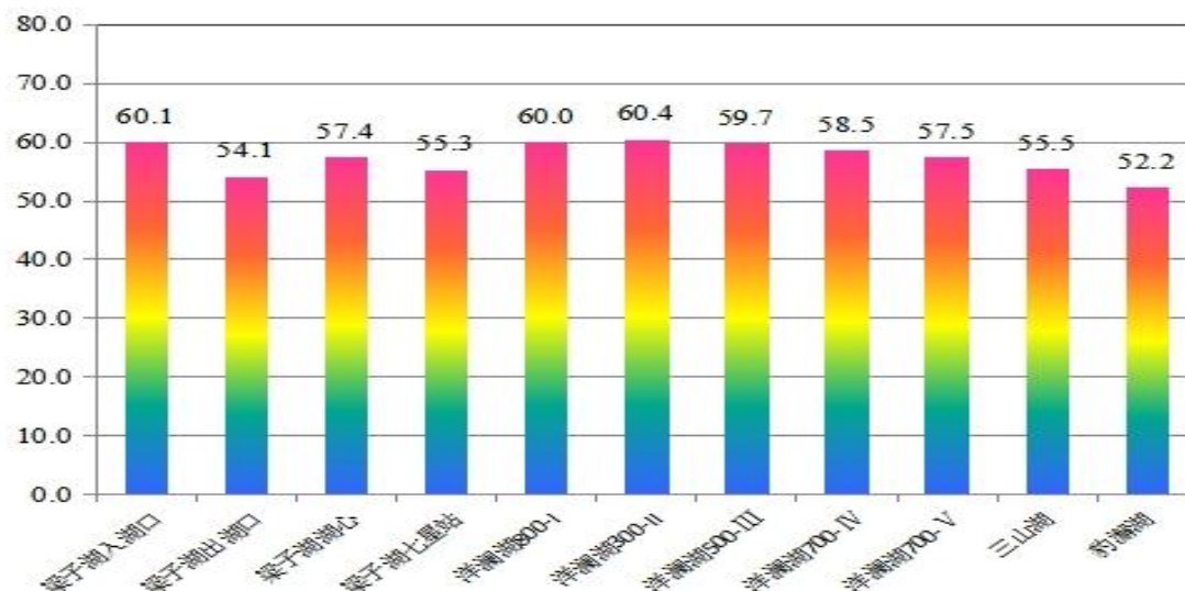
图4 梁子湖、洋澜湖、三山湖、豹澥湖营养指数图
