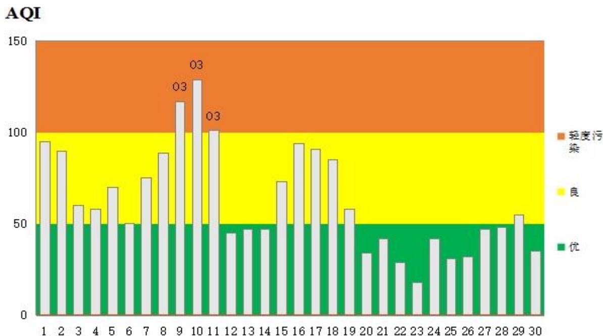
图 2 2023 年 9 月鄂州市区空气质量指数分布图
