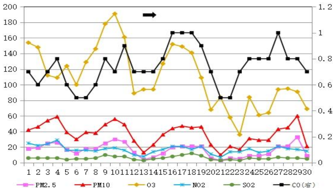
图1 9月份鄂州市城区六项污染物日浓度变化趋势
