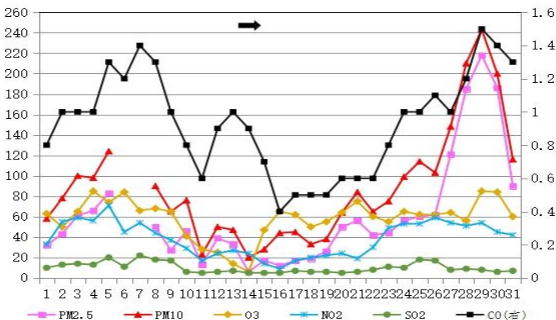
图 1 12 月份鄂州市城区六项污染物日浓度变化趋势
