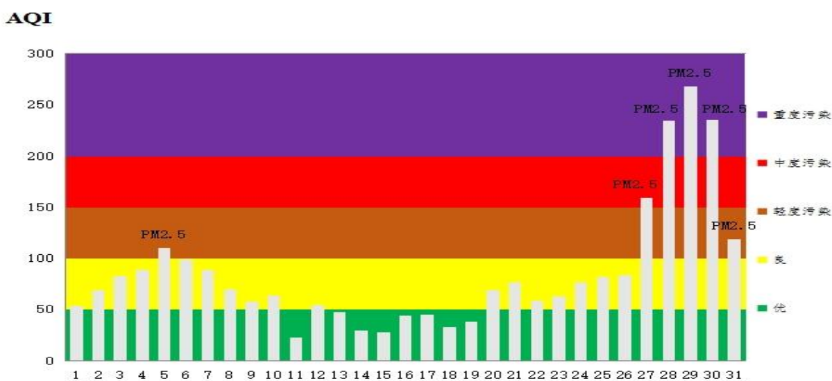
图 2 2023 年 12 月鄂州市区空气质量指数分布图
