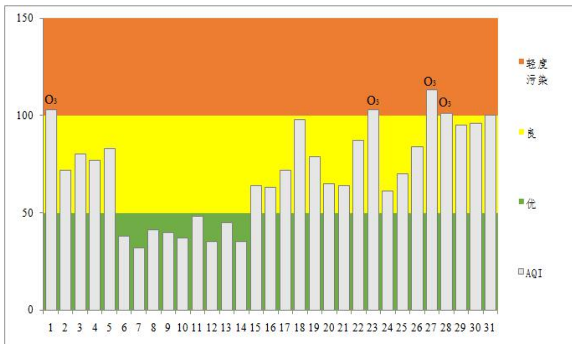
图2 2020年8月鄂州市区空气质量指数及超标天首要污染物分布图
