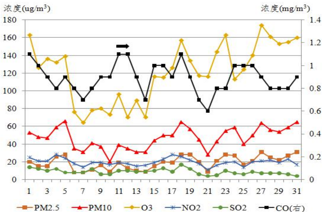
图1 8月份鄂州市城区六项污染物日浓度变化趋势
