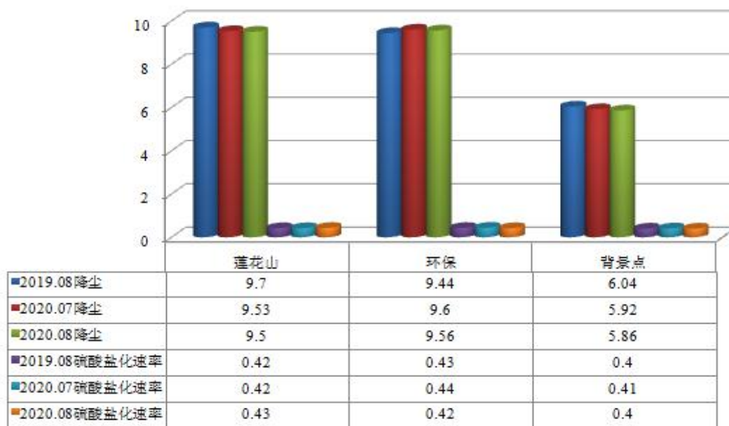
图5：城区8月降尘及硫酸盐化速率
