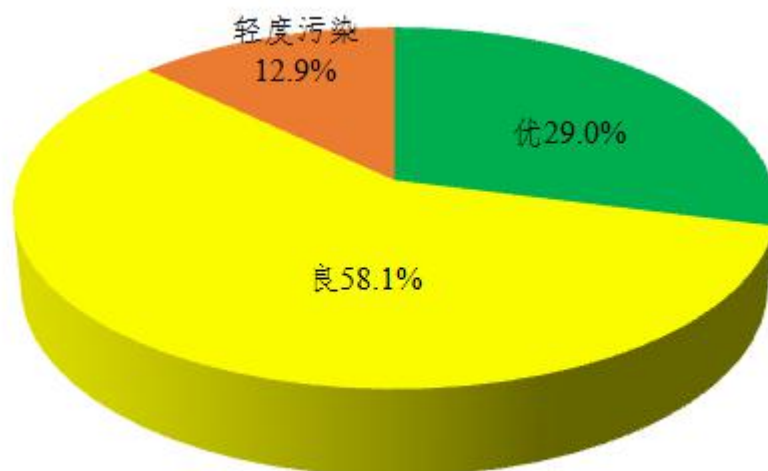
图3 2020年8月鄂州市区空气质量比例图
