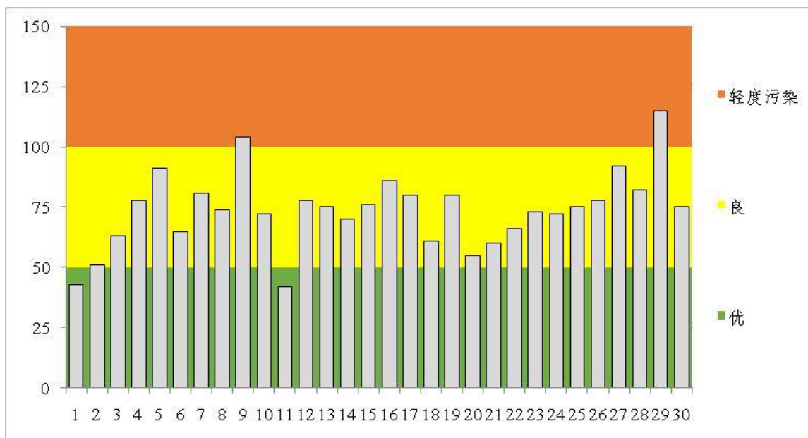
图2: 4月鄂州市区空气质量指数及超标天首要污染物分布图
