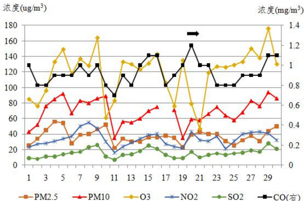
图1 4月份鄂州市城区六项污染物日浓度变化趋势
