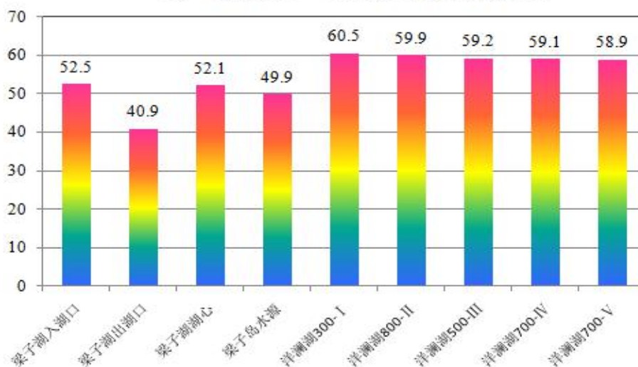
图4 梁子湖、洋澜湖营养指数图
