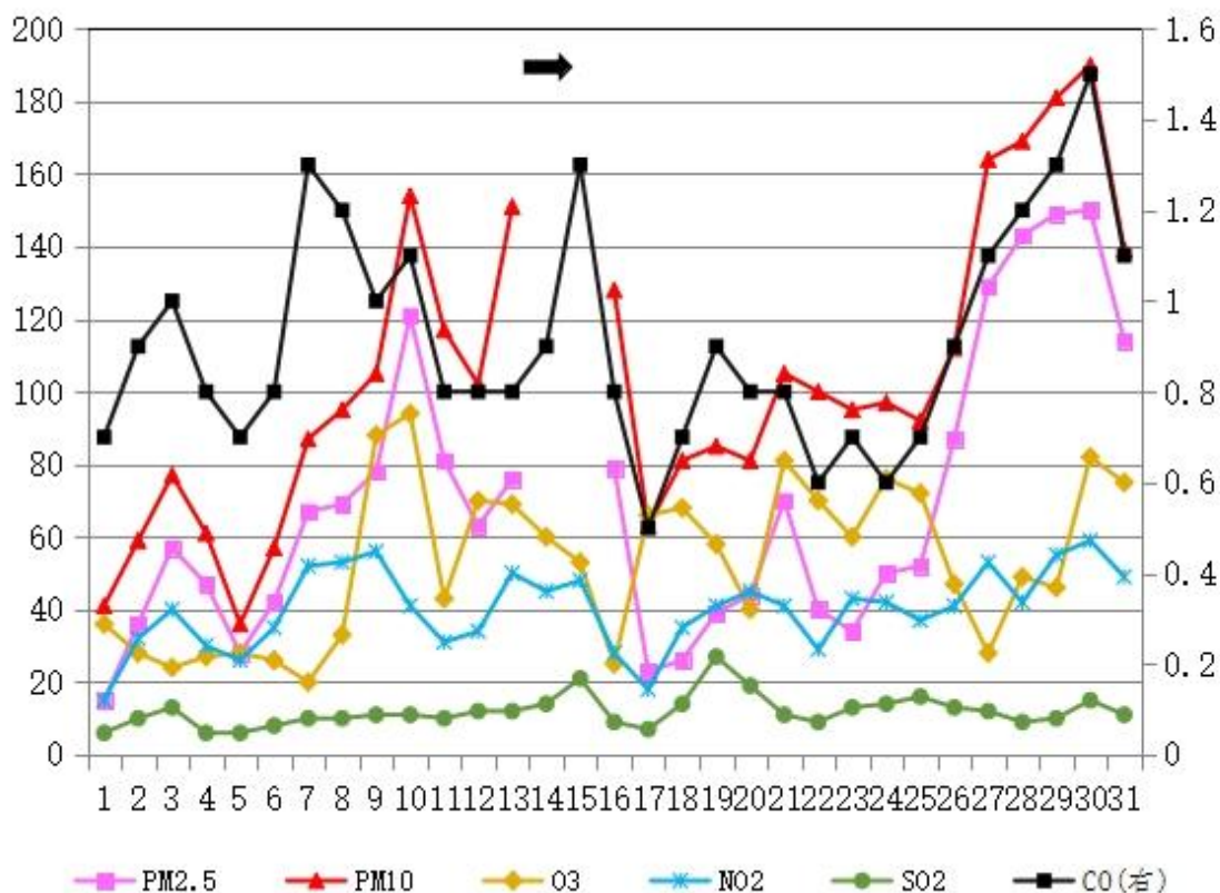
图 1 12 月份鄂州市城区六项污染物日浓度变化趋势
