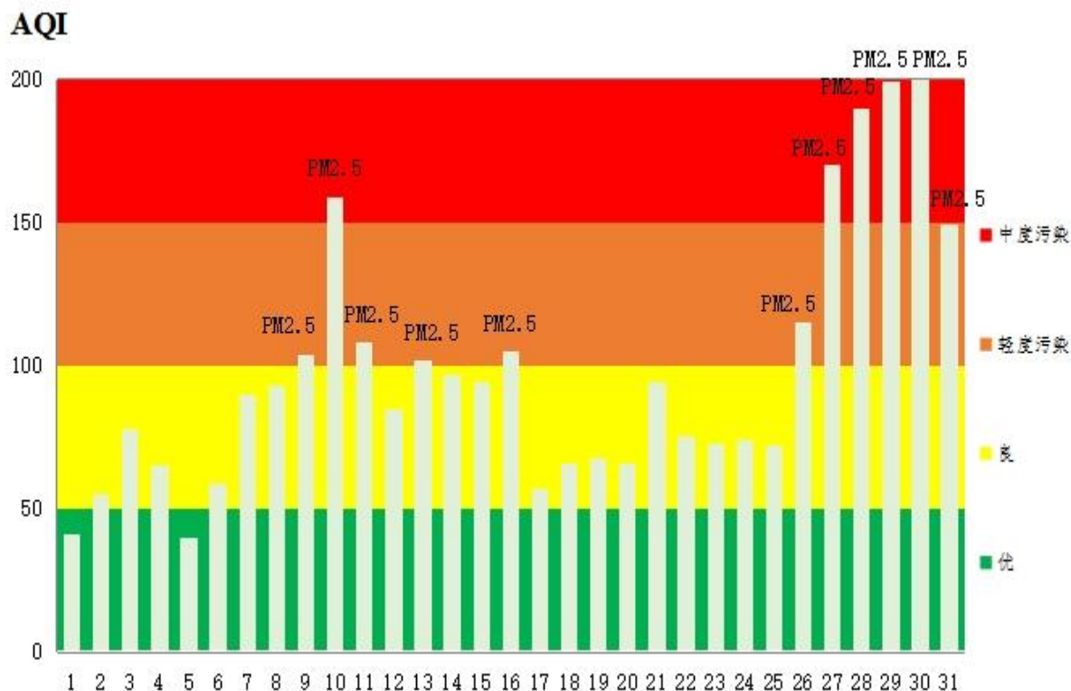
图 2 2022 年 12 月鄂州市区空气质量指数分布图
