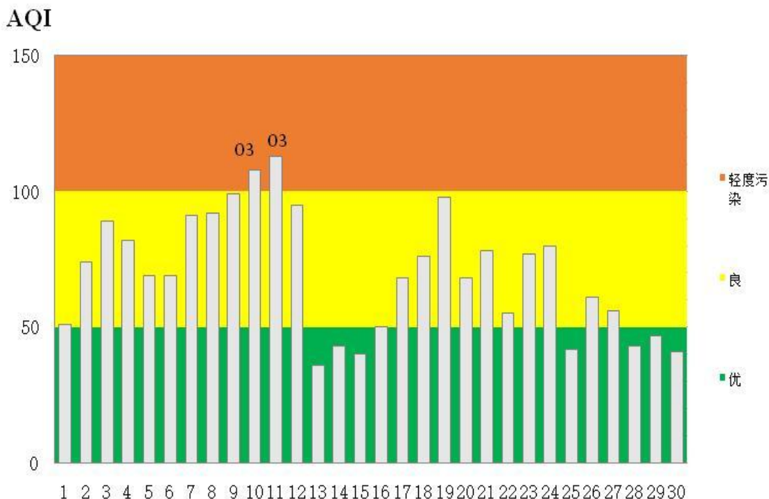
图 2 2022 年 4 月鄂州市区空气质量指数分布图
