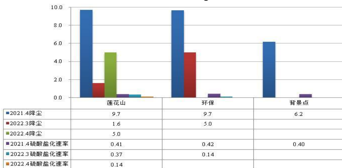
图 5 城区 4 月降尘及硫酸盐化速率
