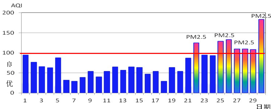
图2 11月份空气质量指数图
