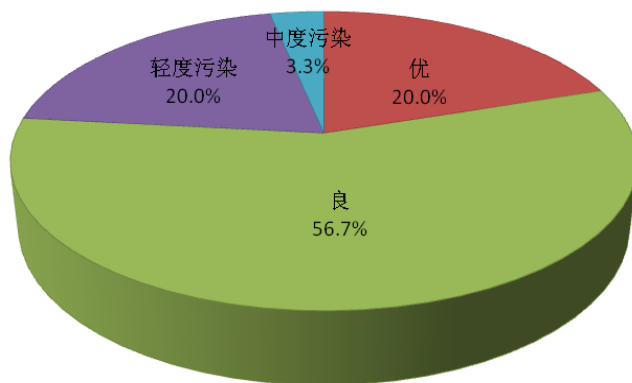
图1 空气质量比例图
