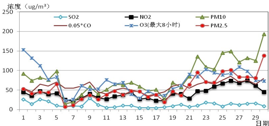
图3 11月份市区大气污染物日均浓度变化曲线图
