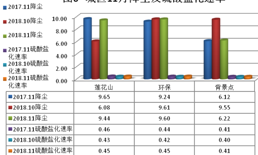
图6 城区11月降尘及硫酸盐化速率
