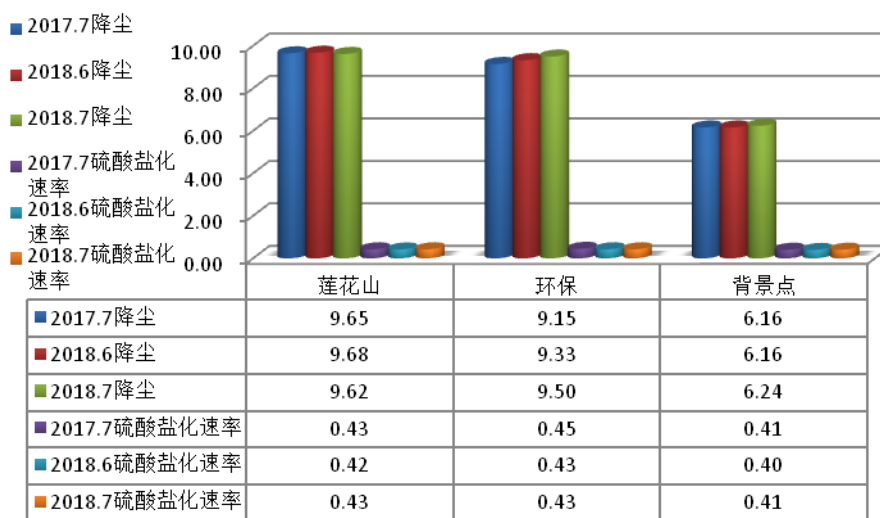
图6 城区7月降尘及硫酸盐化速率
