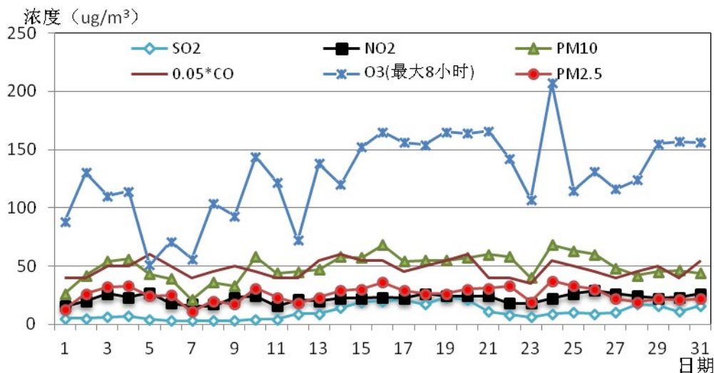
图3 七月份市区大气污染物日均浓度变化曲线图
