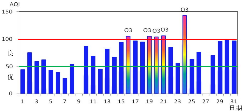
图2 七月份空气质量指数图
