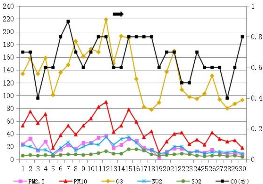
图1 6月份鄂州市城区六项污染物日浓度变化趋势
