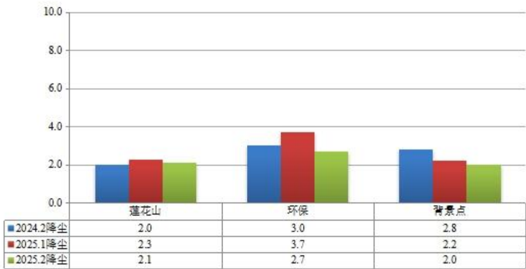
图 5 城区 2 月降尘
